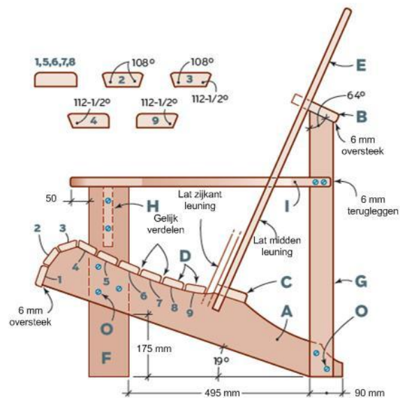
Dwarsdoorsnede
