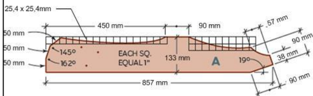
Zijkant zitting
